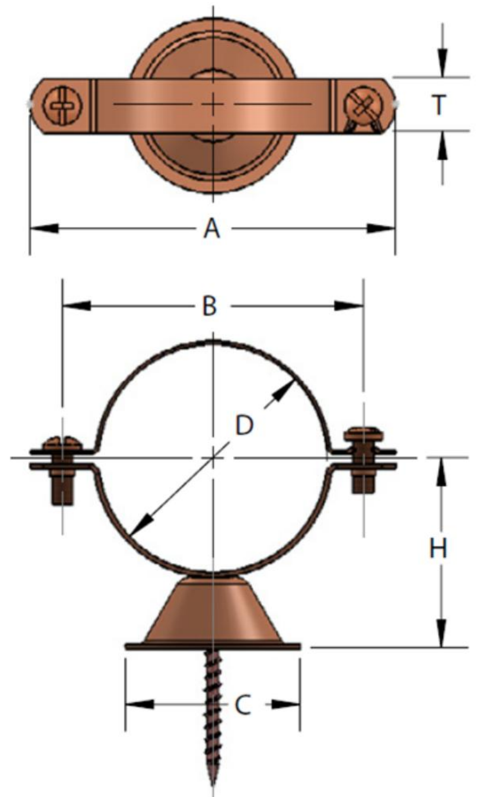
FIG. 129CT VAN (BELL TYPE) HANGER FOR COPPER TUBE
